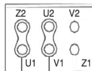
Conexión para Sentido de Giro Antihorario
